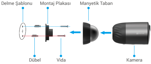
Şekil 1 Manyetik Tabanla Monte Etme
