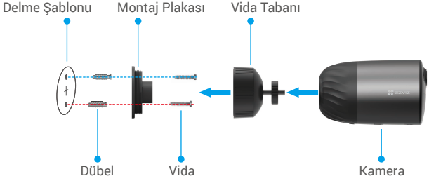
Şekil 2 Vida Tabanı ile Monte Etme
